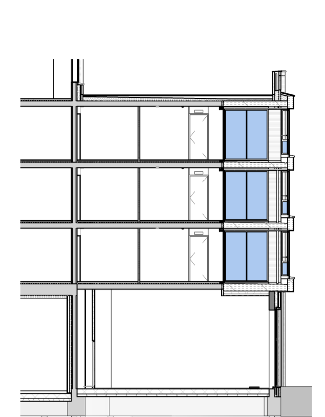
doorsnede A pand I schaal 1:200
