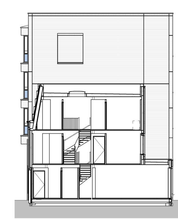
zijgevel pand I (boven E) schaal 1:200
