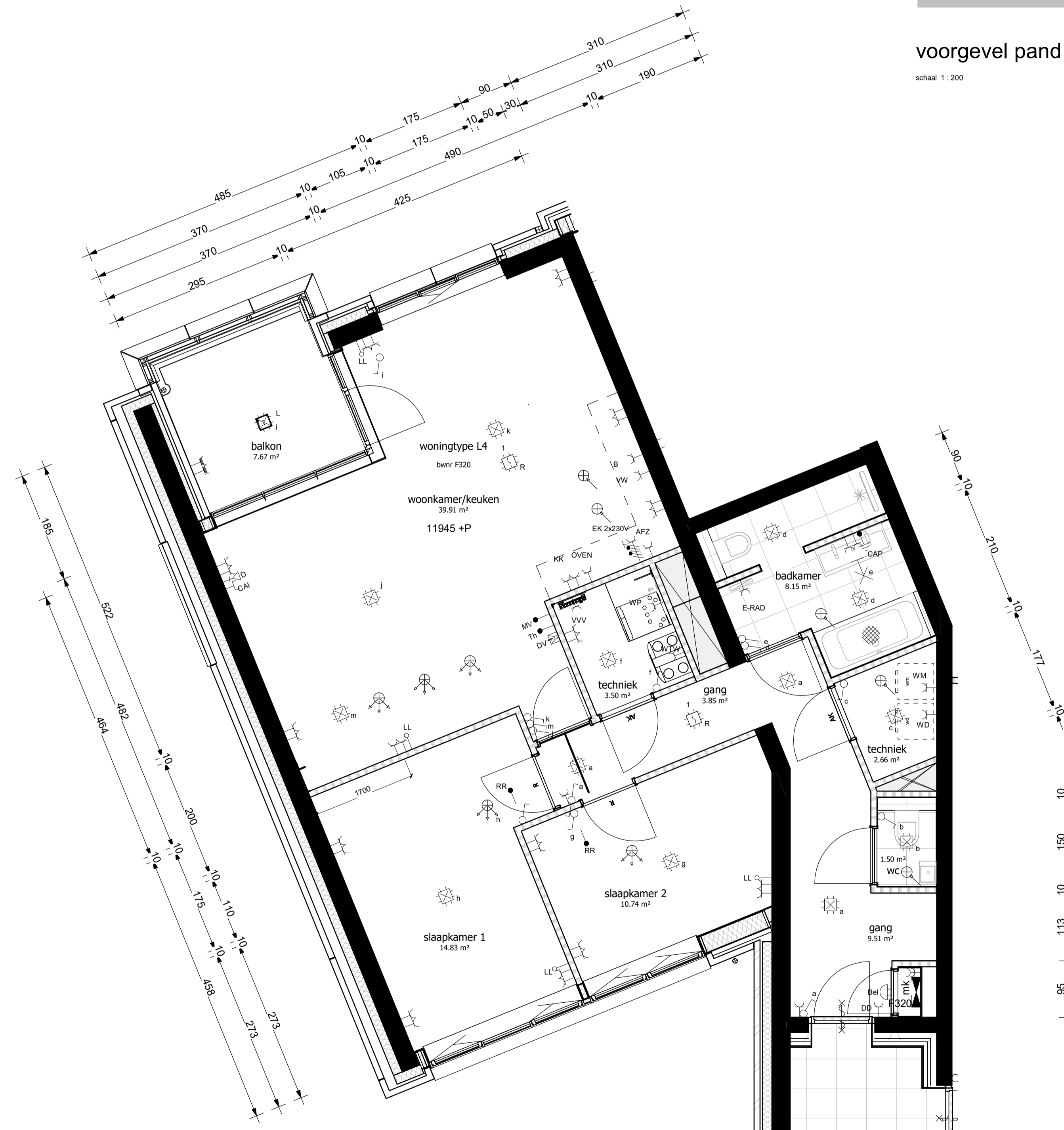
bouwnummer F320
