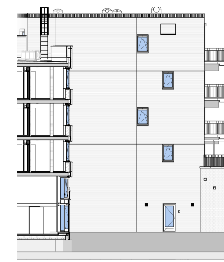
Zijgevel pand H schaal 1:200
