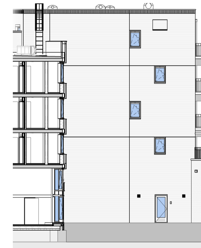
Zijgevel pand H
