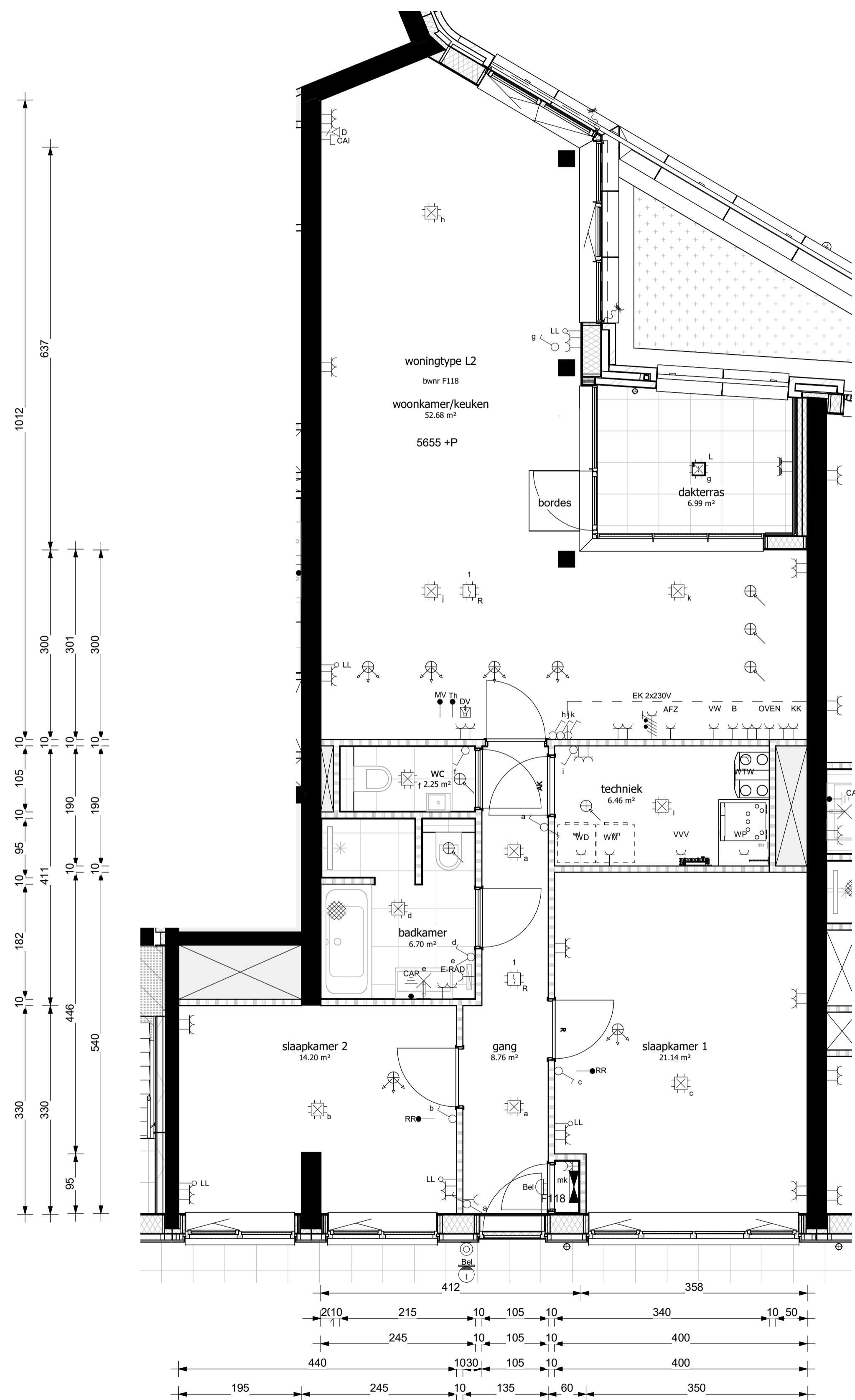
bouwnummer F118 schaal 1:50
