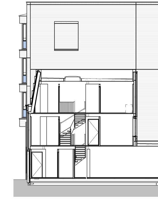
zijgevel pand I (boven E)
