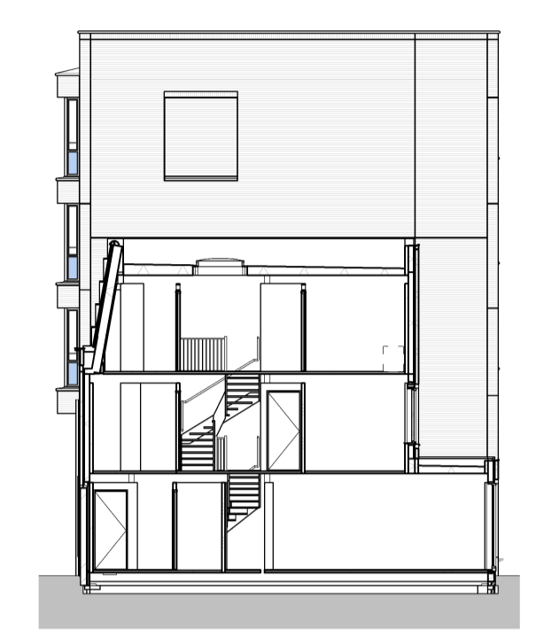
zijgevel pand I (boven E) schaal 1:200
