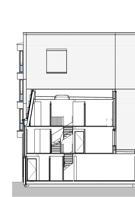
zijgevel pand I (boven E)
