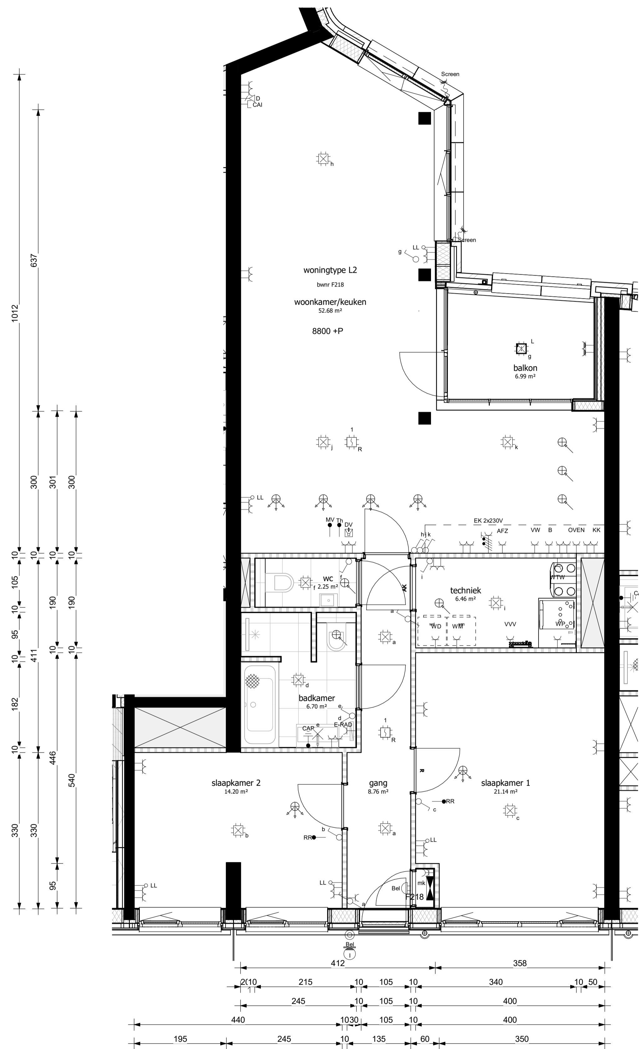
bouwnummer F218 schaal 1:50
