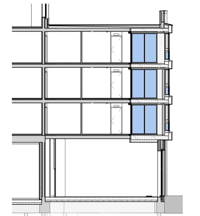
doorsnede A pand I schaal 1:200
