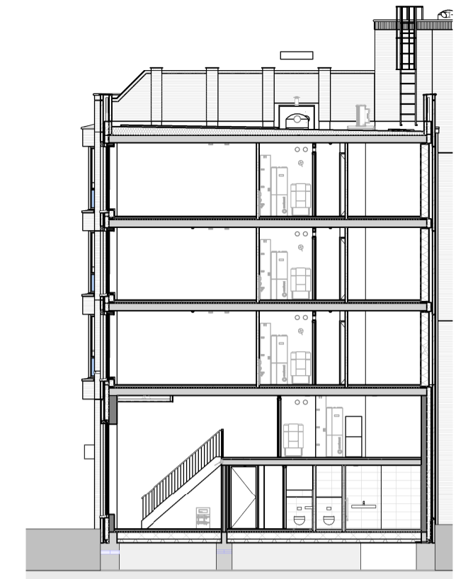
doorsnede B pand I
