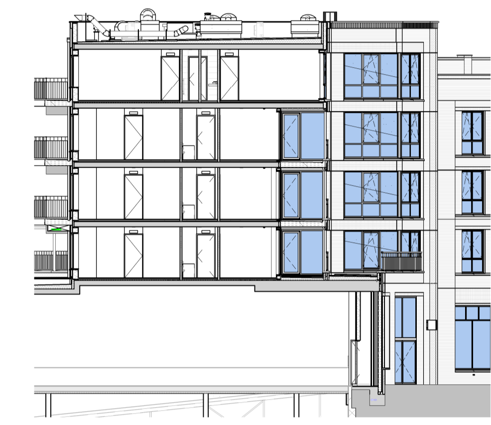
doorsnede B pand H schaal 1:200
