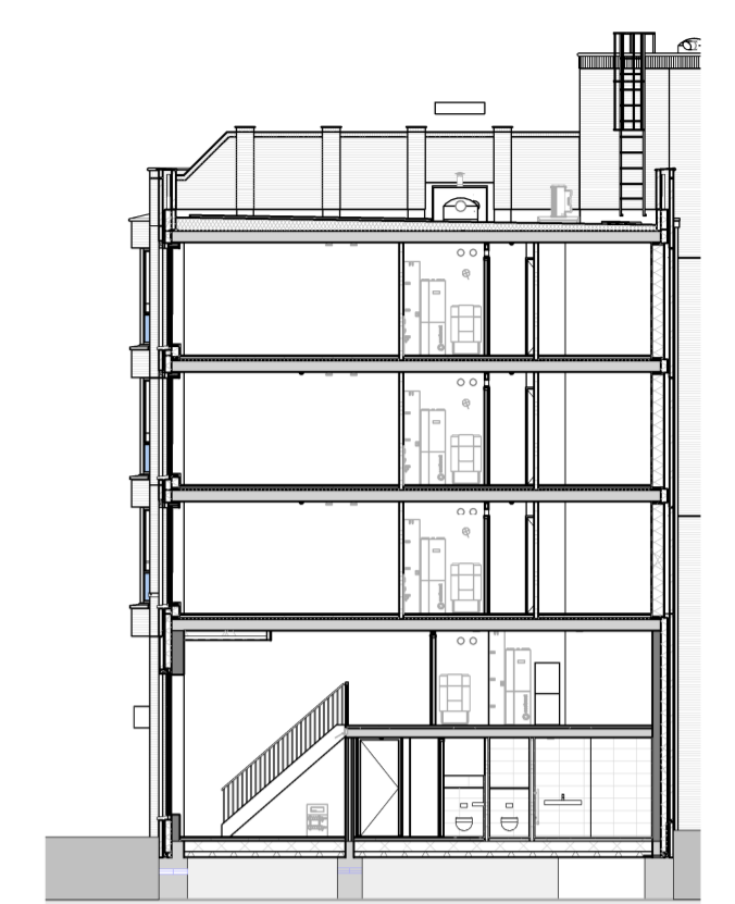
doorsnede B pand I schaal 1:200
