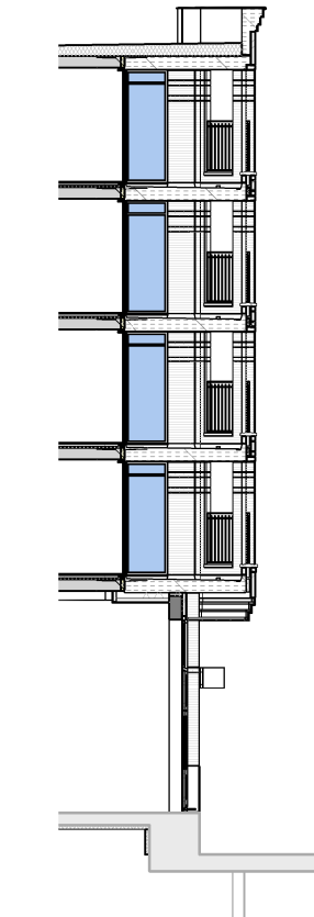
doorsnede pand E (fragment B)
