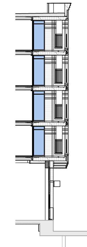
doorsnede pand E (fragment B)
