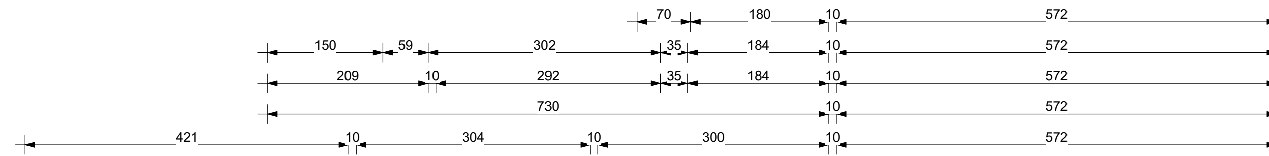
voorgevel pand D
