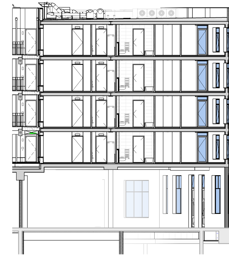
doorsnede pand E (fragment A)
