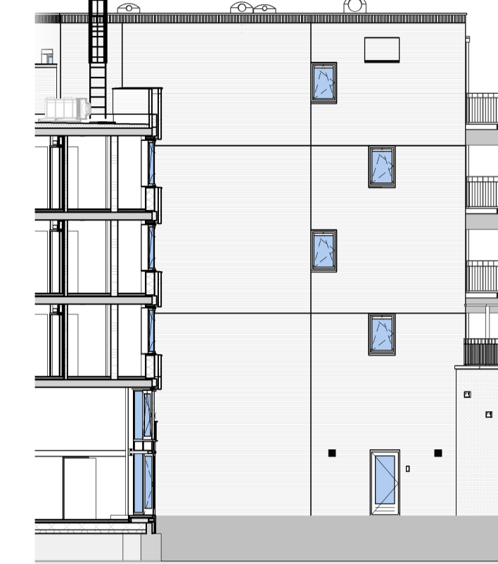
zijgevel pand H
