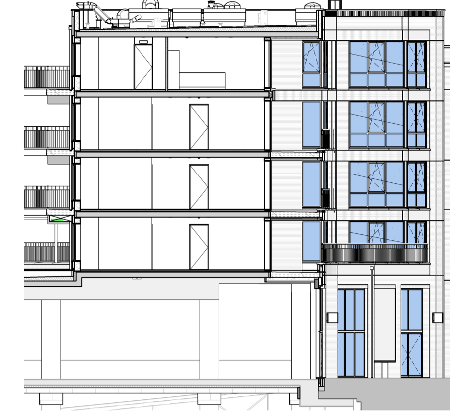
doorsnede A pand H
