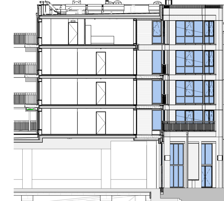
doorsnede A pand G
