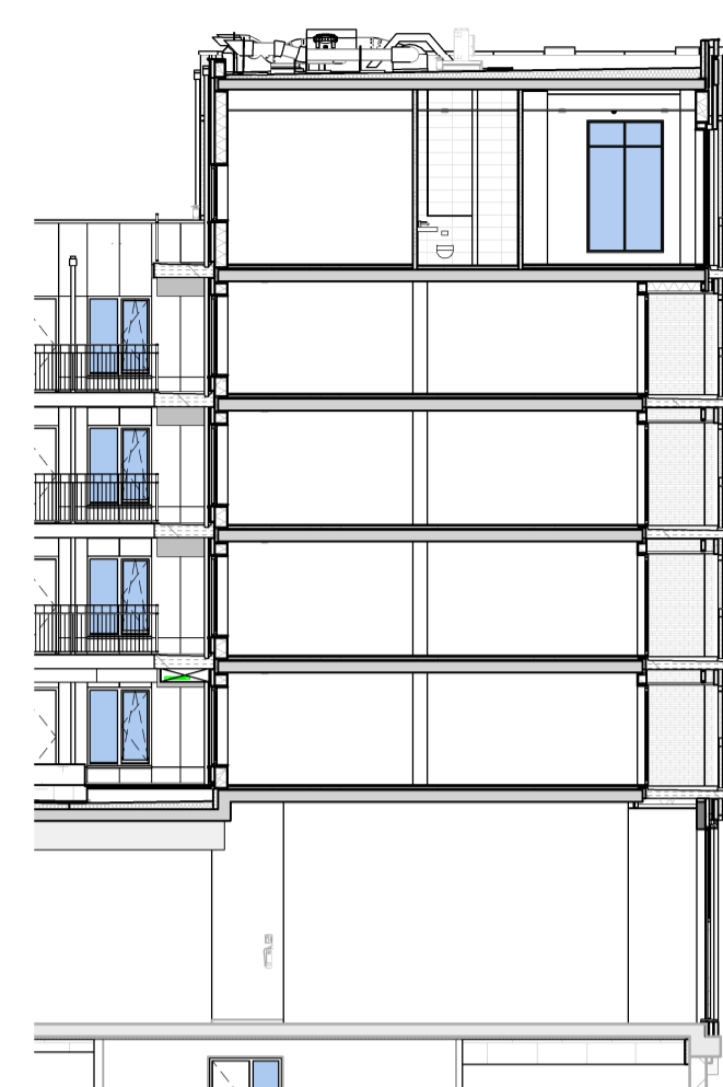
doorsnede C
