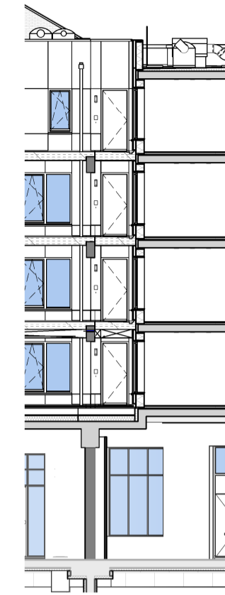
achtergevel pand F
