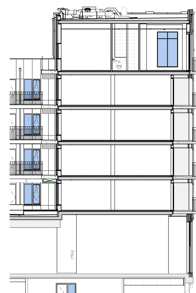
doorsnede C
