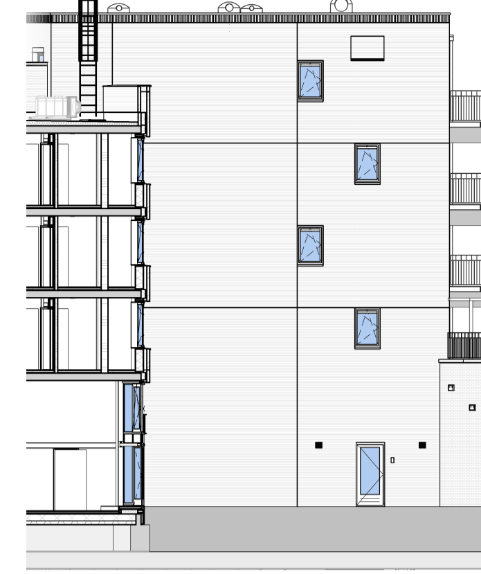
zijgevel pand H
