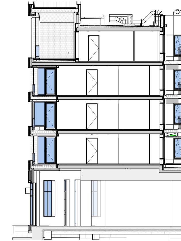
doorsnede A pand G
