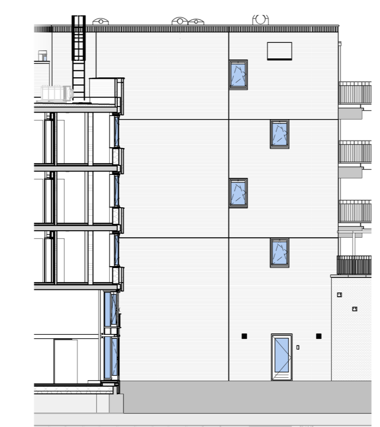
zijgevel pand H schaal 1:200
