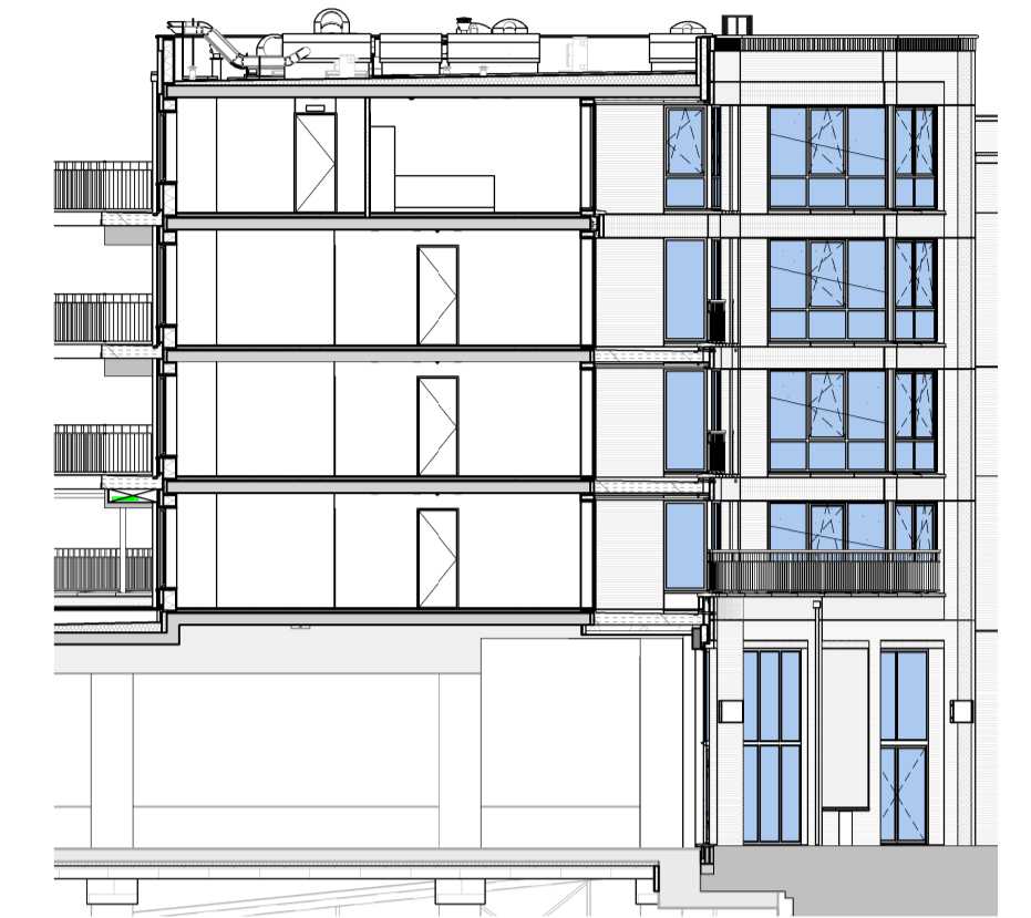
doorsnede A pand H
