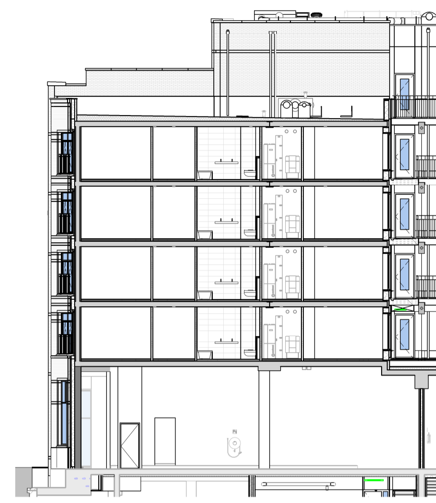
achtergevel pand D
